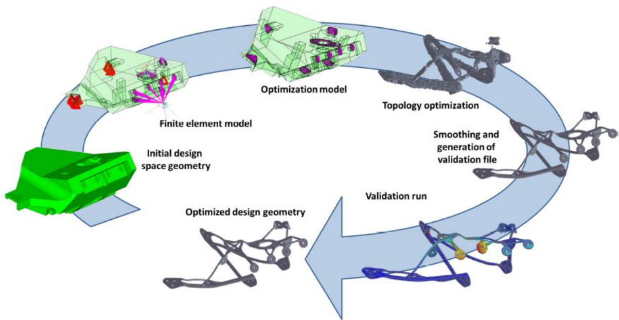
Figuur 1: Ontwerpcyclus van de topologische optimalisatie
