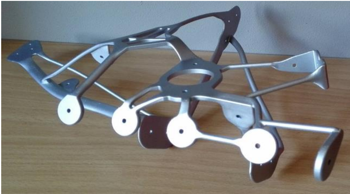
Figuur 5: 3D-geprinte draagstructuur
