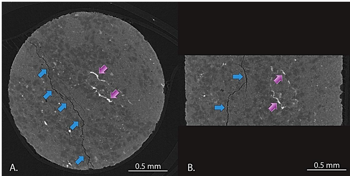
Figuur 1: CT-beelden van een fijnkorrelige zandsteen gekarakteriseerd door fossiele structuren (paarse pijlen) en breuken (blauwe pijlen). Deze beelden hebben een resolutie van 2.8 \mu\text{m} .
