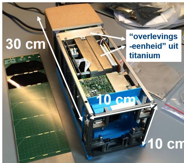
Figuur 3: Geassembleerde satelliet voor de testcampagne met 2 zichtbaar gemonteerde "overlevingseenheden"
