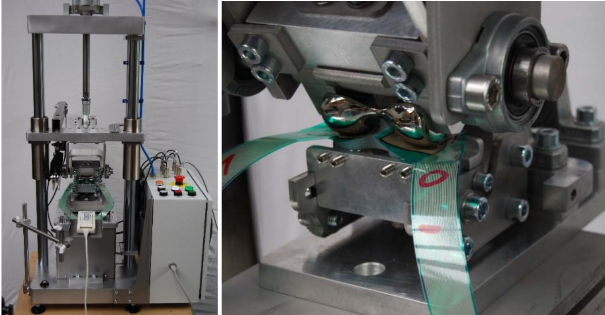
Figuur 1: Proefstand
