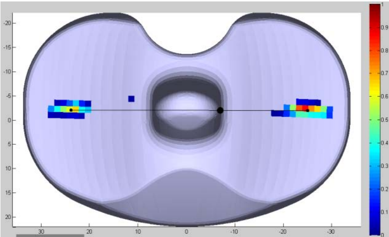
Figuur 2: Visualisatie drukmeting
